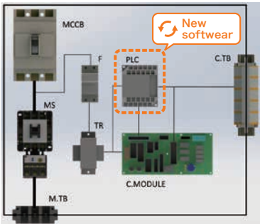
Unit inside configuration ユニット内部構成図
